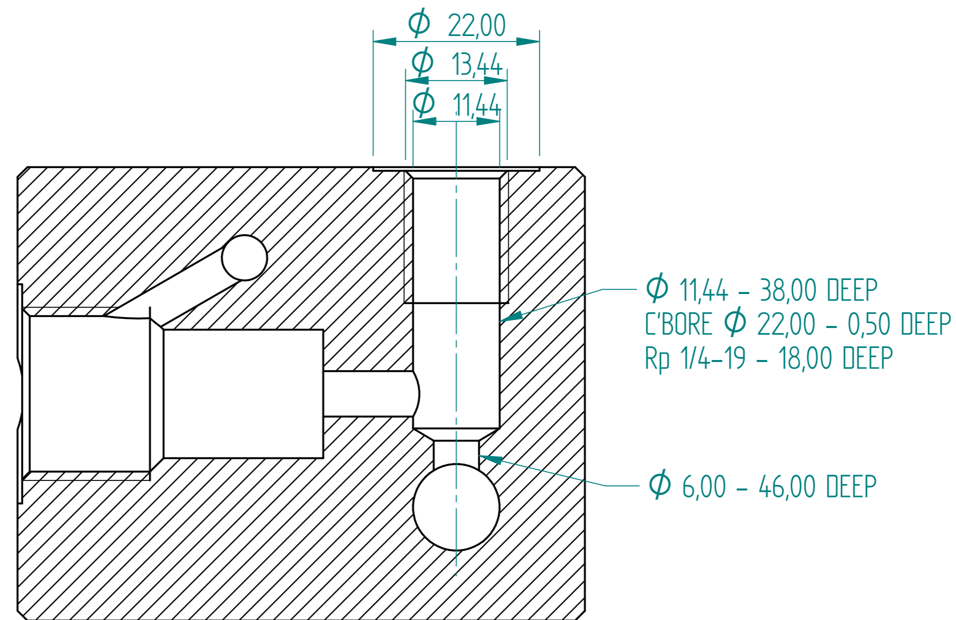
SECTION D-D
